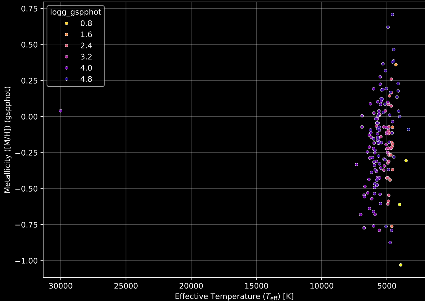
APOGEE DR17 Field: [273-35-O_TESS] Stellar Population Parameters (n= 163)
